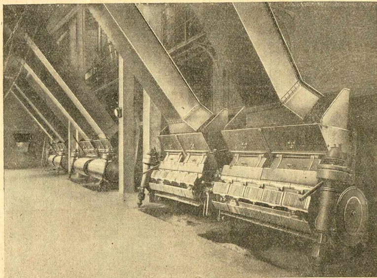
Générateurs multitubulaires à flux direct produisant chacun 8.000 kg. de vapeur à l'heure installés aux Houillères de Montrambert et de la Béraudière
